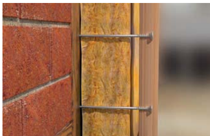
Abstandsmontagen
